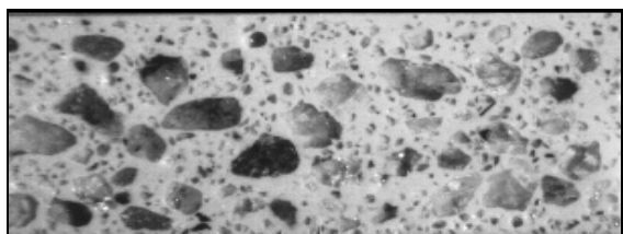
Genomskärning av NM Golv 100
